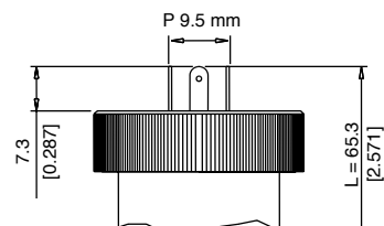
M - 4 pole connector EN 175301-803C
