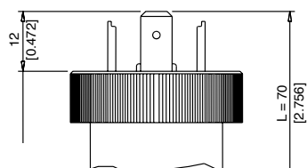
E - 4 pole connector EN 175301-803A
